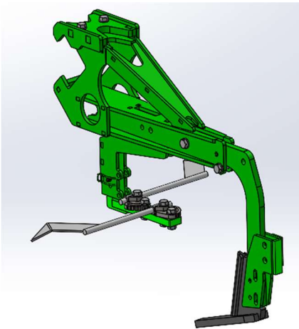
Hackelement vorne
