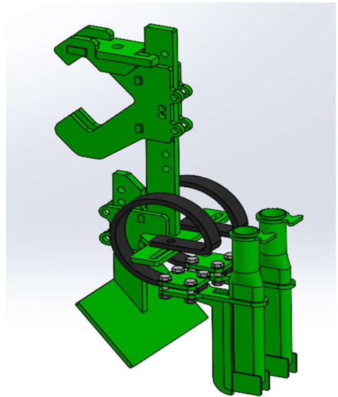
Breitstreubalken
