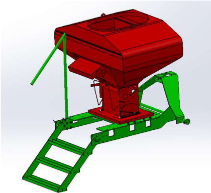
Sämaschinenaufbau
